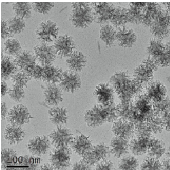
图2 单分散介孔纳米二氧化硅纳米微球（星状）TEM
