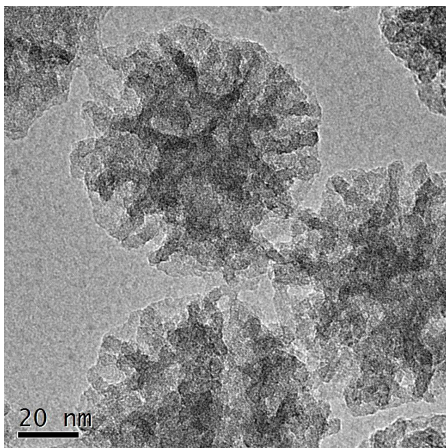
图3 单分散介孔纳米二氧化硅纳米微球（星状）TEM
